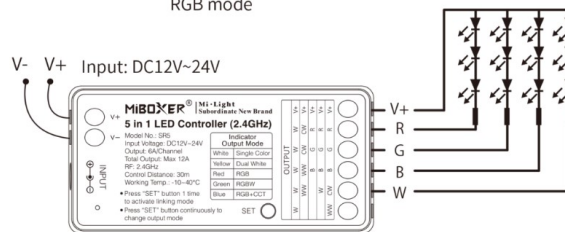
RGB mode
