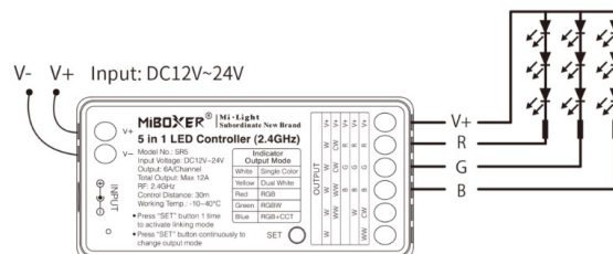
RGB mode
